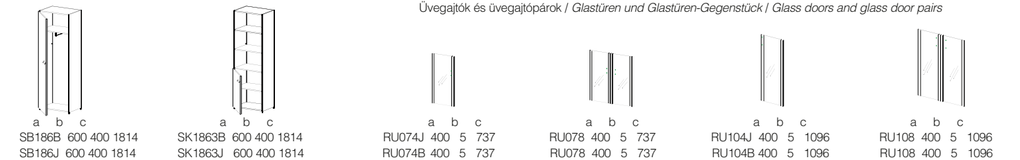
Üvegajtók és üvegajtópárok / Glastüren und Glastüren-Gegenstück / Glass doors and glass door pairs
