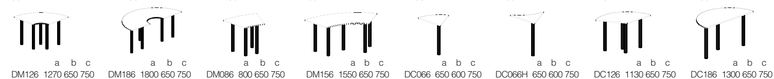
65 cm-es elemek / 65 cm Elemente / 65 cm elements 90° 180° 30° 60° 60° 60° 120° 180°
