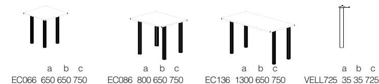
Tárgyalók / Besprechungstische / Meeting tables
